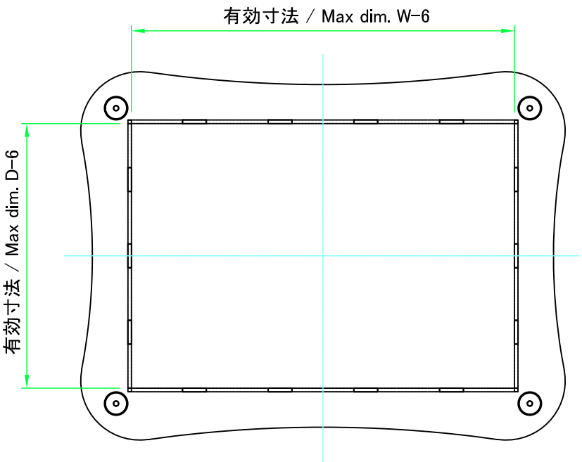
下カバー / Bottom cover
